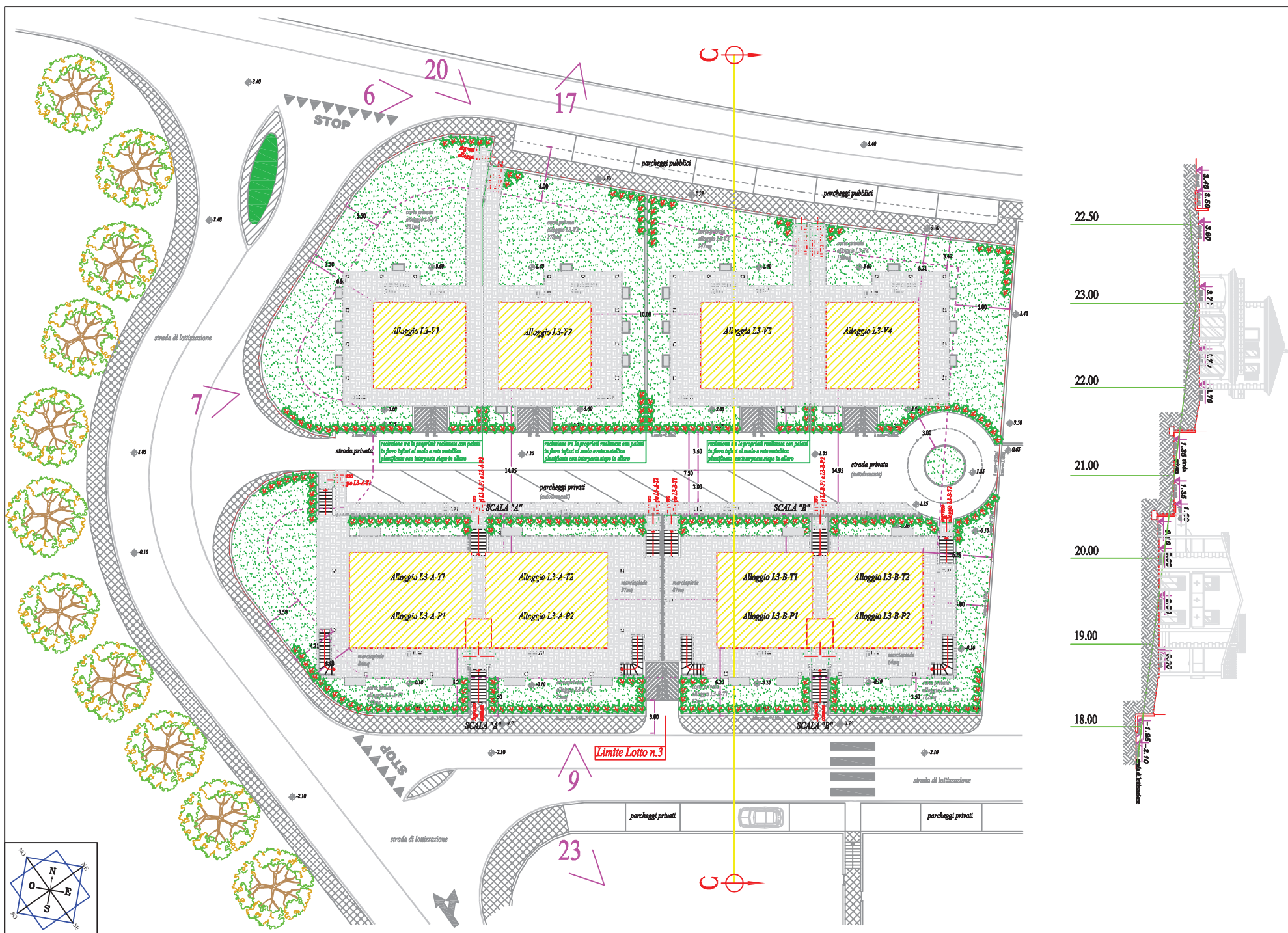
PLANIMETRIA GENERALE LOTTO N.3 e PROFILO DEL TERRENO Sezione C-C (scala 1:200)
