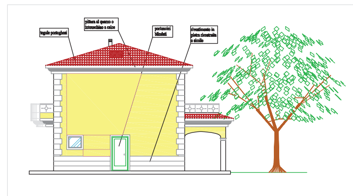
Prospetto Est-NordEst
