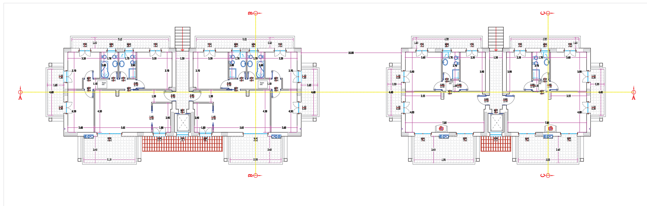
Piano primo
