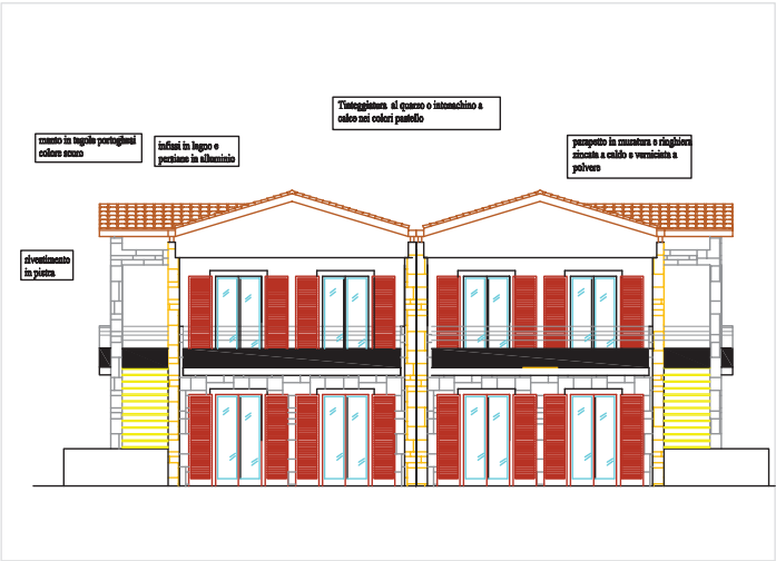
Prospetto Nord-NordOvest
