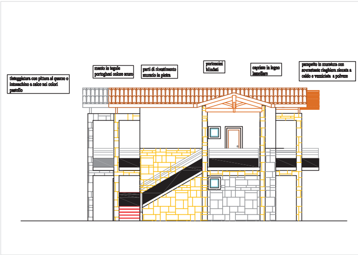
Prospetto Laterale
